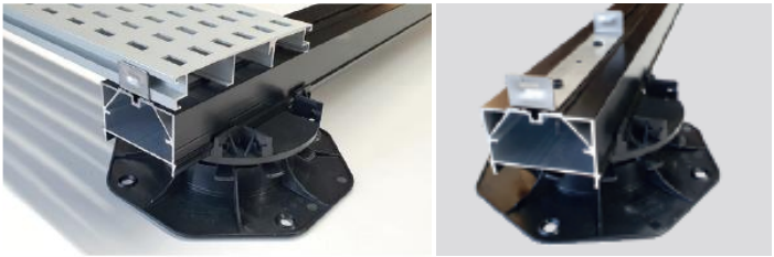
Drainage- und Belüftungsprofil Montageklammer
